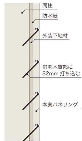
【図1】本実パネリングの取付施工
